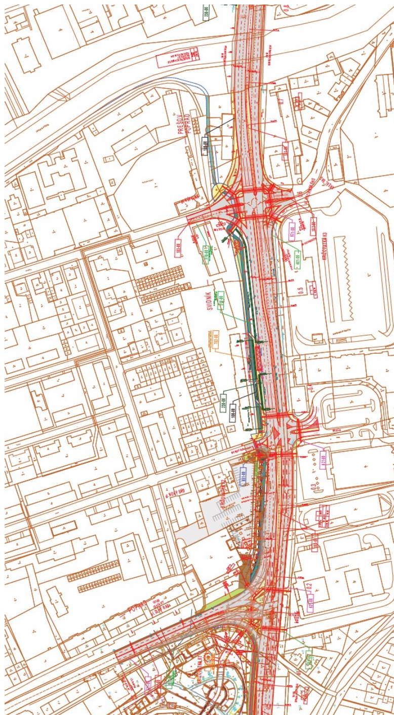
Situácia: Cyklochodník na ul. Slovenská v Bardejov
